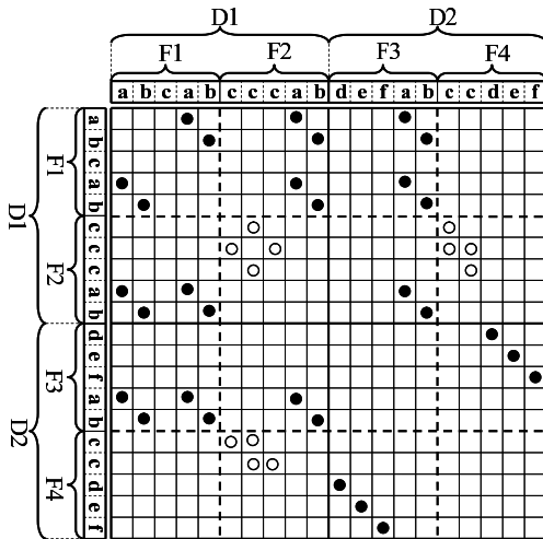
F1, F2, F3, F4: ファイル D1, D2: ディレクトリ ●: RNRが閾値以上のコードクローンに含まれるトークン ○: RNRが閾値未満のコードクローンに含まれるトークン
