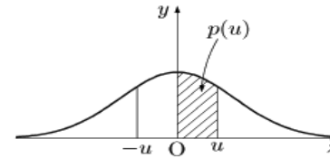
正 規 分 布 表
