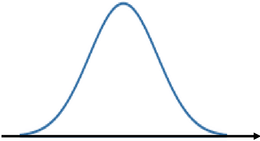
図 正規分布のグラフ
