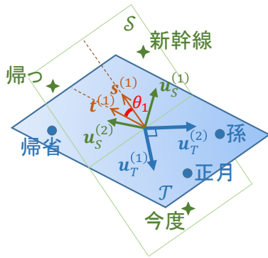
図 1 メッセージ「今度、新幹線で帰っておいで」の部分空間 \mathcal{S} と、キーワード（「正月」、「帰省」、「孫」、…）を設定した宛先の部分空間 \mathcal{T} の間の類似度評価。 \mathcal{S} と \mathcal{T} の基底ベクトルはそれぞれ \mathbf{U}_S = [\mathbf{u}_S^{(1)}, \mathbf{u}_S^{(2)}] \mathbf{U}_T = [\mathbf{u}_T^{(1)}, \mathbf{u}_T^{(2)}] である。 \mathcal{S} と \mathcal{T} の第 1 正準ベクトル \mathbf{s}^{(1)} と \mathbf{t}^{(1)} のなす第 1 正準角 \theta_1 が小さいほど類似度が高い。
